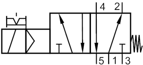
1 x 5/2-luistiventtiili (limittämätön) monostabiili
