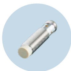
Detectores inductivos Robusta carcasa de acero inoxidable para el sector alimentario
