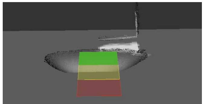
O obstáculo na frente do veículo é projetado em uma imagem no solo. Uma das três zonas ou a área na chamada matriz de ocupação é então indicada como ocupada.
