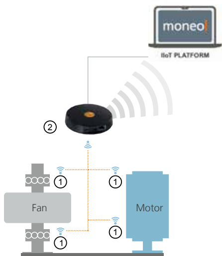
1) VW Vibration sensor 2) ZB0929 Gateway 3) moneo|RTM
